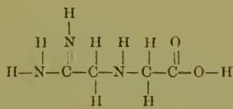
Methyluramido-Essigsäure (Kreatin).
